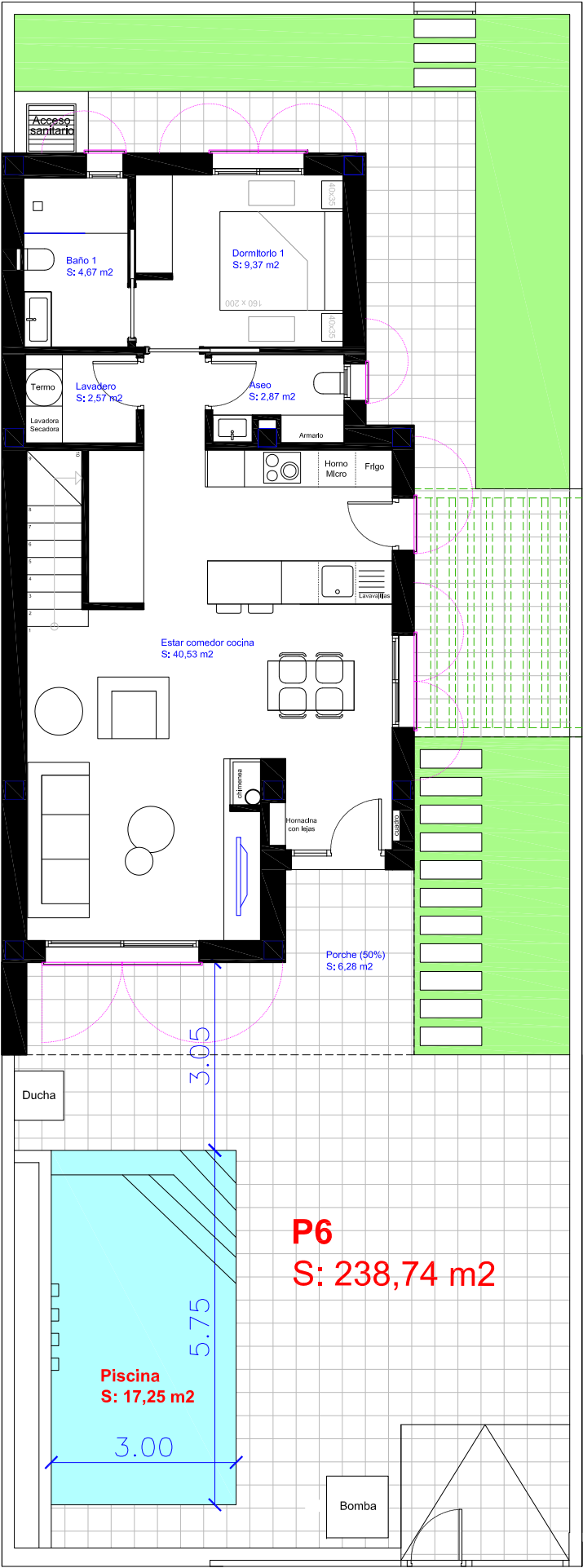
Planta baja
